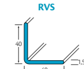
Gelijkzijdig hoekprofiel Art.nr.: 518/rvs Lengte 3 m 1
