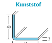
Gelijkzijdig hoekprofiel Art.nr.: 518/ks Lengte 3 m 1
