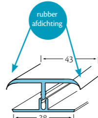
2-delige verbingsprofiel Art.nr.: 1022 Lengte 3 m 1
